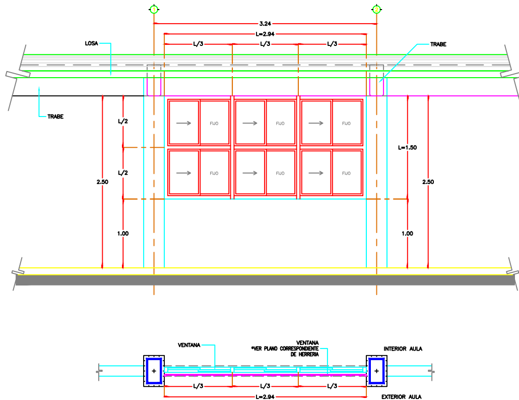
CANCELERIA EN FACHADA POSTERIOR – MUROS BAJOS
