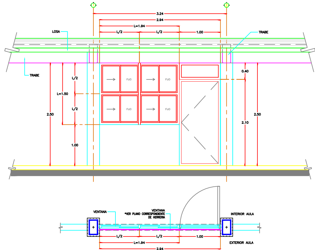
CANCELERIA EN FACHADA PRINCIPAL – MUROS BAJOS
