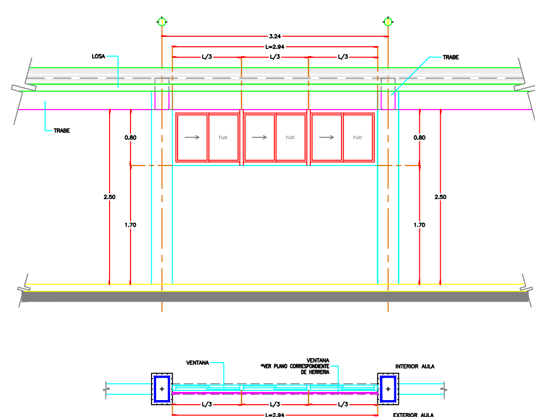
CANCELERIA EN FACHADA POSTERIOR – MUROS ALTOS
