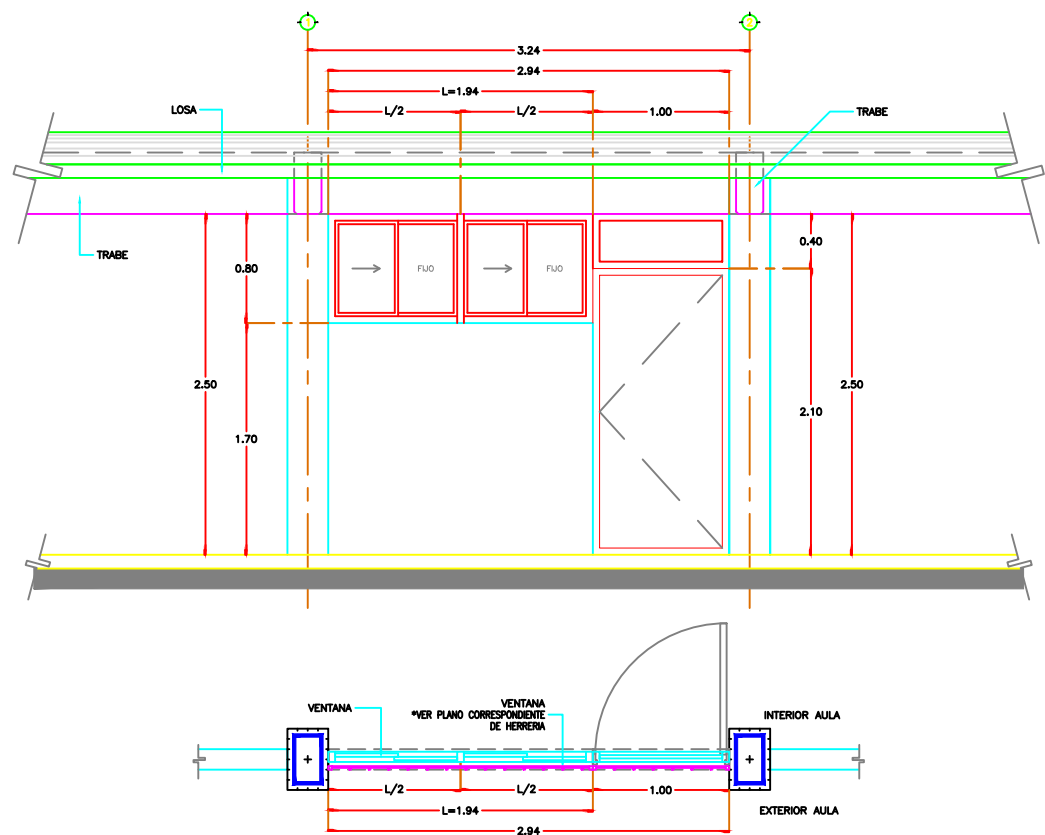
CANCELERIA EN FACHADA PRINCIPAL – MUROS ALTOS
