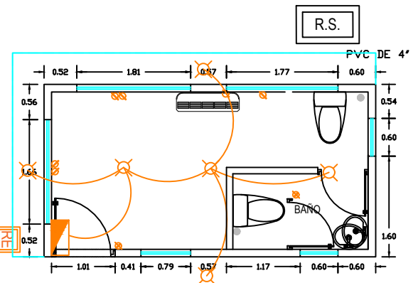
PLANTA ELECTRICA
