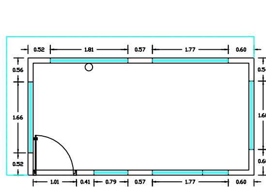
PLANTA ACTUAL
