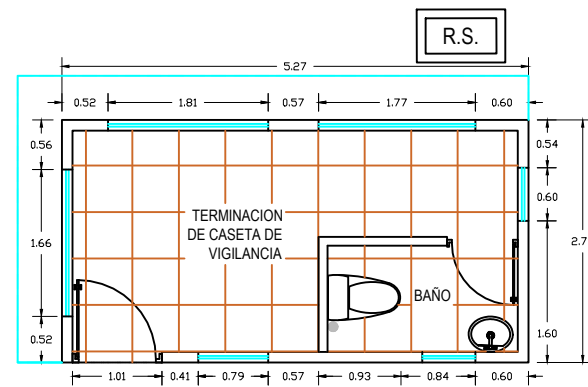
PLANTA PROPUESTA
