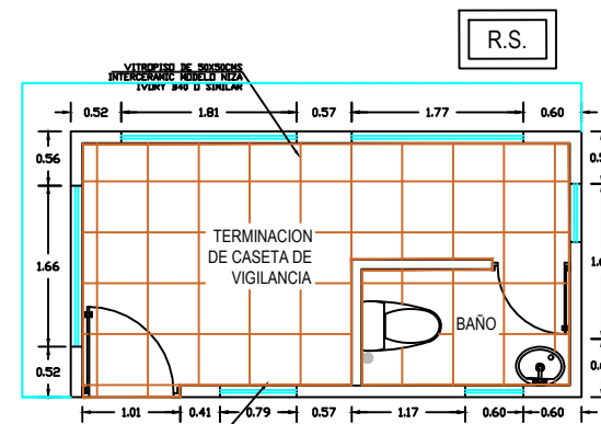
PLANTA PISO
