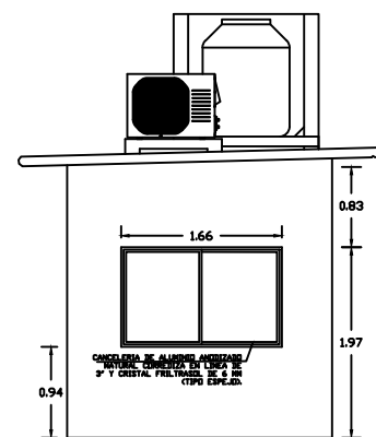
FACHADA LATERAL
