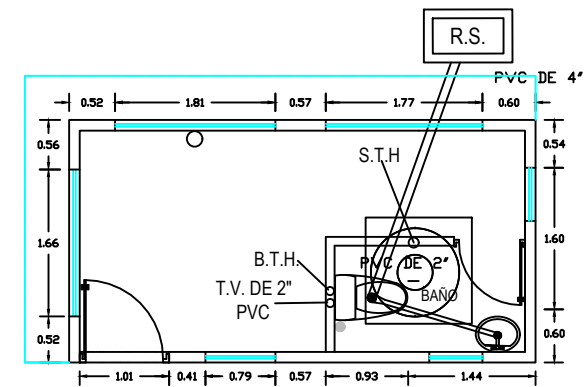
INST. HIDRAULICA INST.SANITARIA
