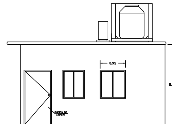
FACHADA POSTERIOR
