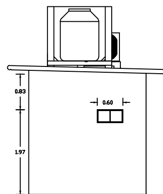
FACHADA LATERAL 1
