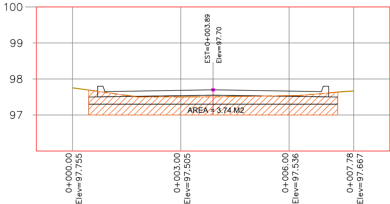
PERFIL 0+080
