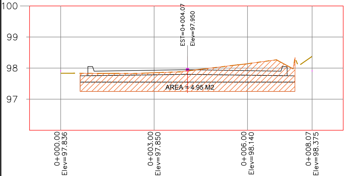
PERFIL 0+040
