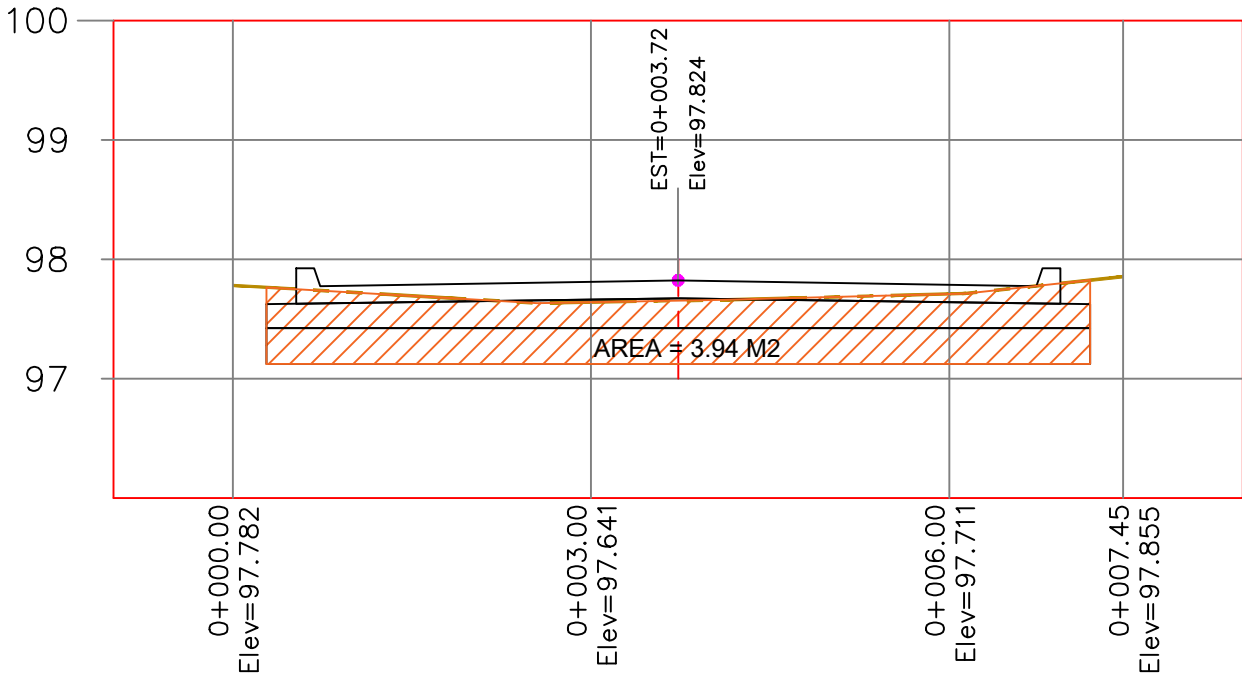
PERFIL 0+060
