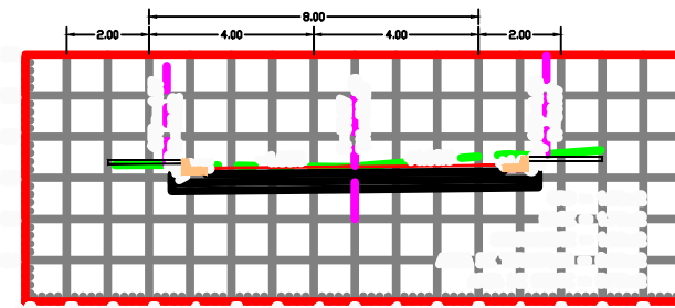
ESTACION 0+090.00
