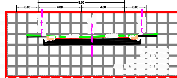
ESTACION 0+120.00
