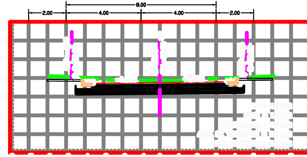
ESTACION 0+080.00
