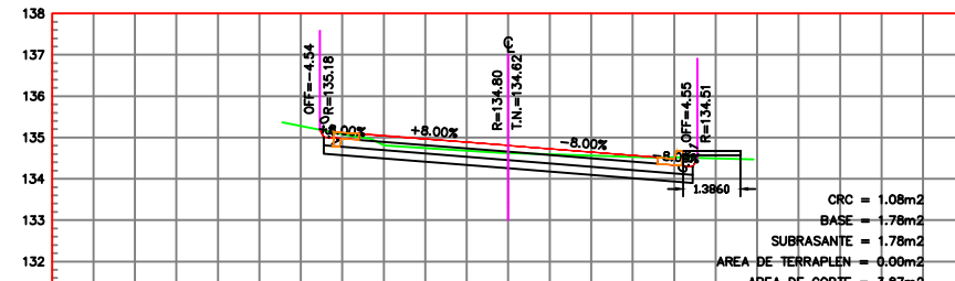
ESTACION 0+095.56 ESCALA HORIZONTAL 1 : 100 ESCALA VERTICAL 1 : 100
