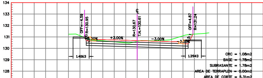
ESTACION 0+010.00 ESCALA HORIZONTAL 1 : 100 ESCALA VERTICAL 1 : 100
