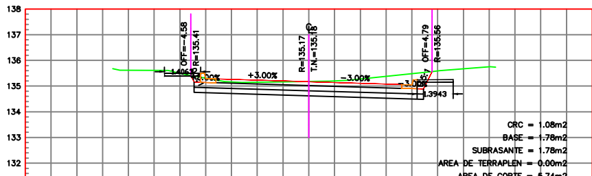
ESTACION 0+040.00 ESCALA HORIZONTAL 1 : 100 ESCALA VERTICAL 1 : 100
