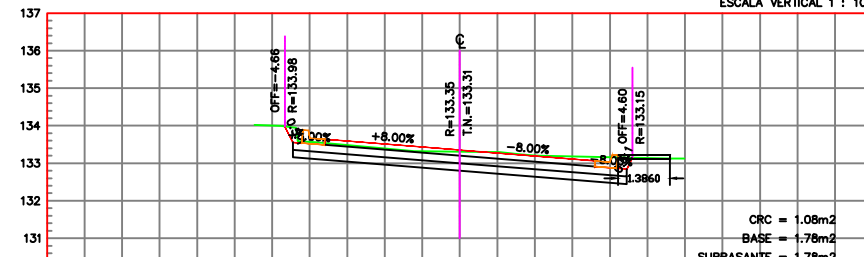
ESTACION 0+107.67 ESCALA HORIZONTAL 1 : 100 ESCALA VERTICAL 1 : 100
