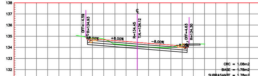
ESTACION 0+100.00 ESCALA HORIZONTAL 1 : 100 ESCALA VERTICAL 1 : 100
