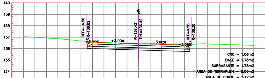
ESTACION 0+070.00 ESCALA HORIZONTAL 1 : 100 ESCALA VERTICAL 1 : 100
