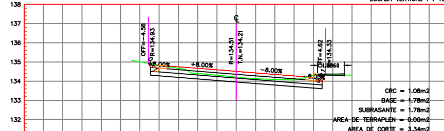
ESTACION 0+099.20 ESCALA HORIZONTAL 1 : 100 ESCALA VERTICAL 1 : 100
