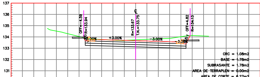
ESTACION 0+030.00 ESCALA HORIZONTAL 1 : 100 ESCALA VERTICAL 1 : 100
