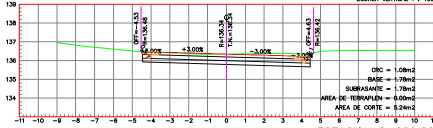
ESTACION 0+060.00 ESCALA HORIZONTAL 1 : 100 ESCALA VERTICAL 1 : 100
