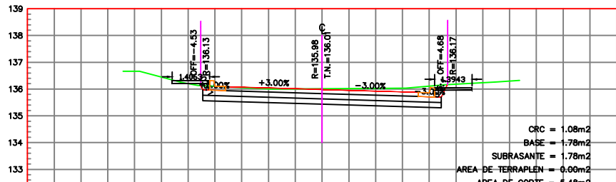
ESTACION 0+050.00 ESCALA HORIZONTAL 1 : 100 ESCALA VERTICAL 1 : 100
