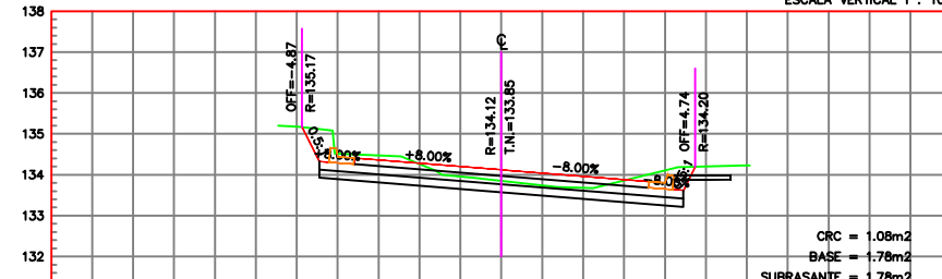
ESTACION 0+102.27 ESCALA HORIZONTAL 1 : 100 ESCALA VERTICAL 1 : 100
