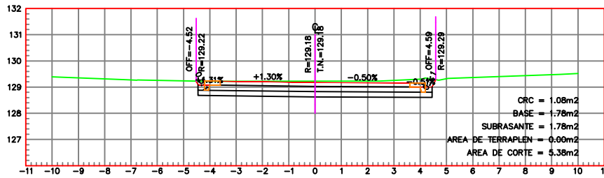
ESTACION 0+00.00 ESCALA HORIZONTAL 1 : 100 ESCALA VERTICAL 1 : 100
