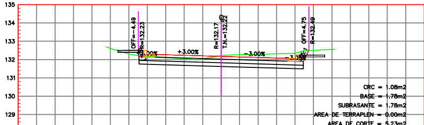
ESTACION 0+020.00 ESCALA HORIZONTAL 1 : 100 ESCALA VERTICAL 1 : 100
