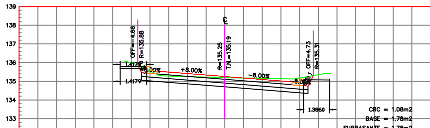
ESTACION 0+090.00 ESCALA HORIZONTAL 1 : 100 ESCALA VERTICAL 1 : 100
