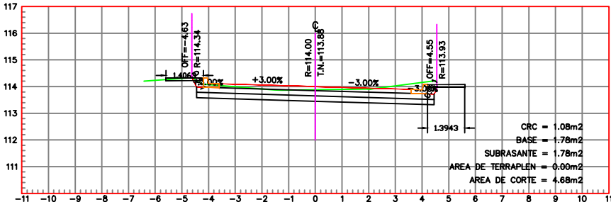
ESTACION 0+220.00 ESCALA HORIZONTAL 1 : 100 ESCALA VERTICAL 1 : 100
