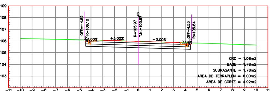
ESTACION 0+275.29 ESCALA HORIZONTAL 1 : 100 ESCALA VERTICAL 1 : 100
