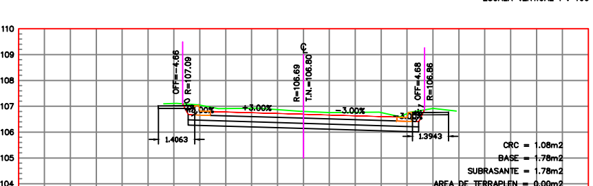
ESTACION 0+270.00 ESCALA HORIZONTAL 1 : 100 ESCALA VERTICAL 1 : 100
