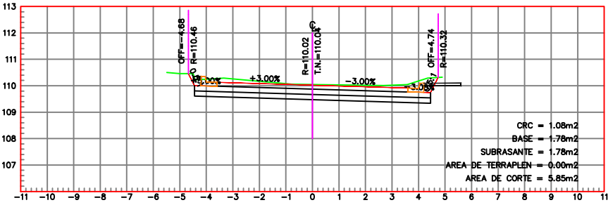
ESTACION 0+245.54 ESCALA HORIZONTAL 1 : 100 ESCALA VERTICAL 1 : 100
