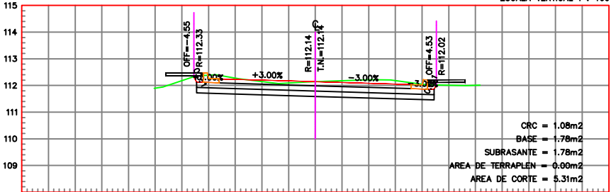
ESTACION 0+230.00 ESCALA HORIZONTAL 1 : 100 ESCALA VERTICAL 1 : 100
