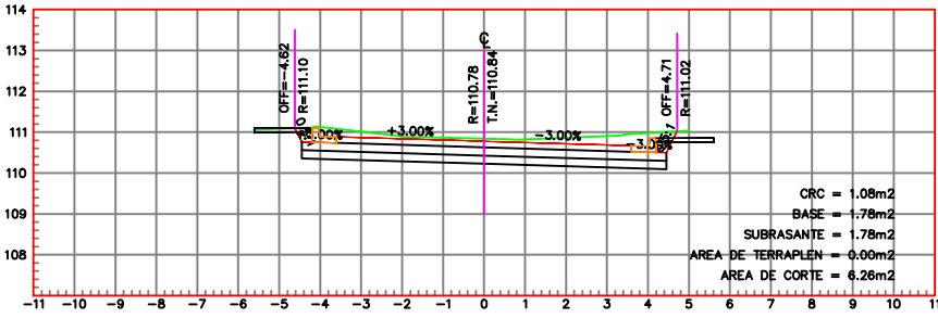
ESTACION 0+240.00 ESCALA HORIZONTAL 1 : 100 ESCALA VERTICAL 1 : 100
