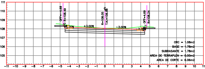
ESTACION 0+260.00 ESCALA HORIZONTAL 1 : 100 ESCALA VERTICAL 1 : 100
