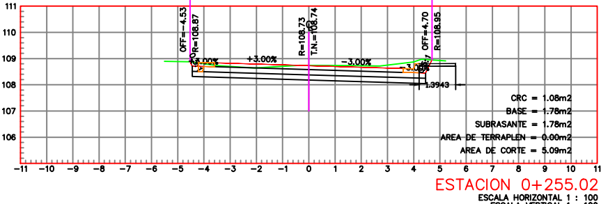
ESTACION 0+255.02 ESCALA HORIZONTAL 1 : 100 ESCALA VERTICAL 1 : 100
