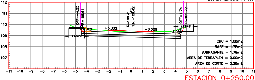
ESTACION 0+250.00 ESCALA HORIZONTAL 1 : 100 ESCALA VERTICAL 1 : 100
