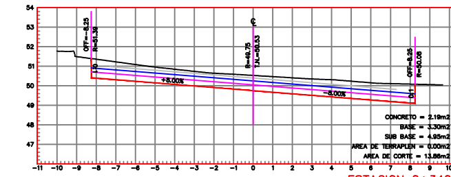
ESTACION 0+340.00 ESCALA HORIZONTAL 1 : 100 ESCALA VERTICAL 1 : 100
