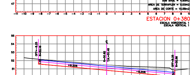
ESTACION 0+400.00 ESCALA HORIZONTAL 1 : 100 ESCALA VERTICAL 1 : 100
