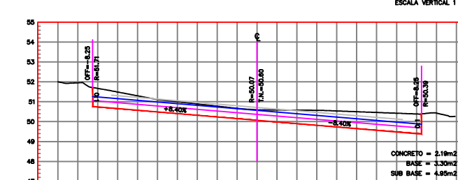
ESTACION 0+360.00 ESCALA HORIZONTAL 1 : 100 ESCALA VERTICAL 1 : 100
