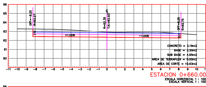
ESTACION 0+660.00 ESCALA HORIZONTAL 1 : 100 ESCALA VERTICAL 1 : 100
