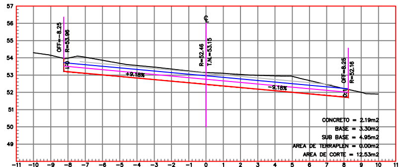
ESTACION 0+460.00 ESCALA HORIZONTAL 1 : 100 ESCALA VERTICAL 1 : 100
