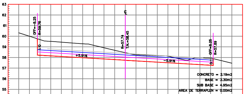
ESTACION 0+540.00 ESCALA HORIZONTAL 1 : 100 ESCALA VERTICAL 1 : 100
