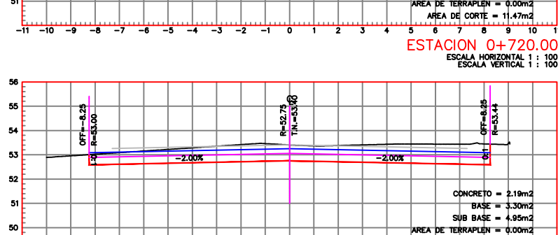
ESTACION 0+720.00 ESCALA HORIZONTAL 1 : 100 ESCALA VERTICAL 1 : 100
