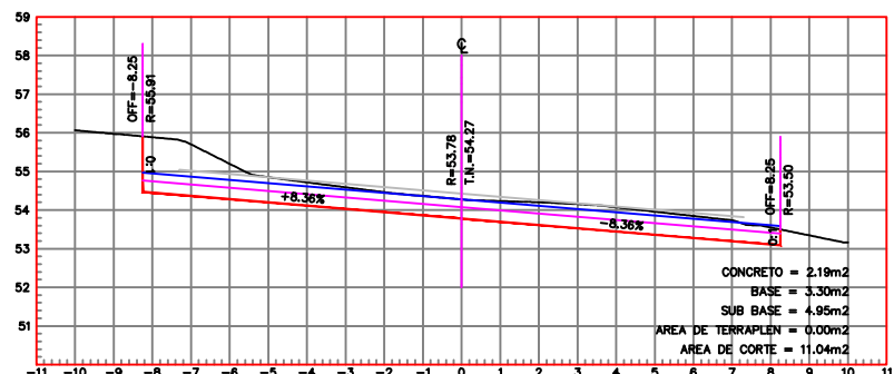
ESTACION 0+480.00 ESCALA HORIZONTAL 1 : 100 ESCALA VERTICAL 1 : 100
