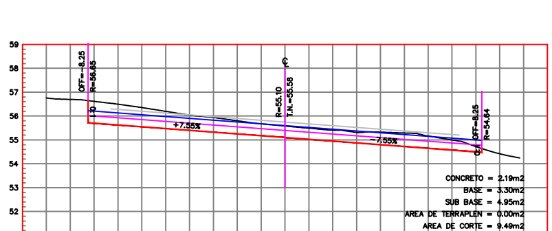
ESTACION 0+500.00 ESCALA HORIZONTAL 1 : 100 ESCALA VERTICAL 1 : 100
