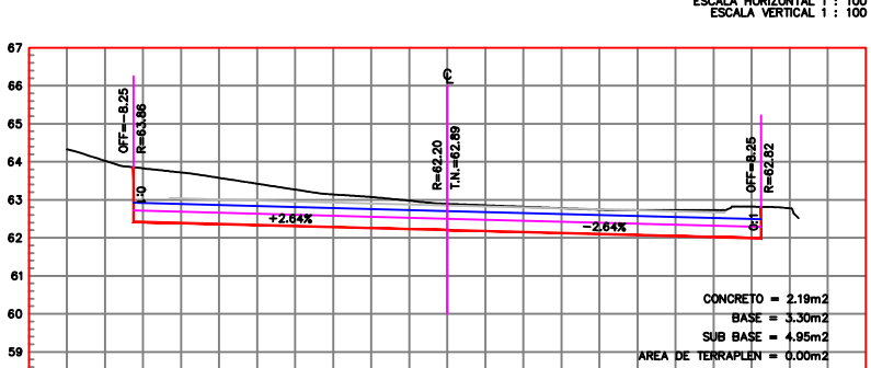
ESTACION 0+620.00 ESCALA HORIZONTAL 1 : 100 ESCALA VERTICAL 1 : 100
