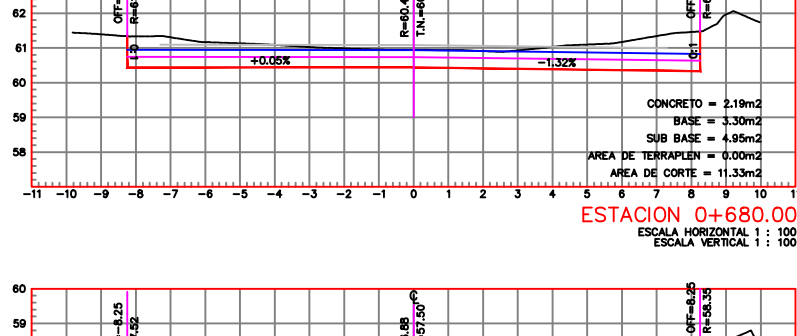
ESTACION 0+680.00 ESCALA HORIZONTAL 1 : 100 ESCALA VERTICAL 1 : 100
