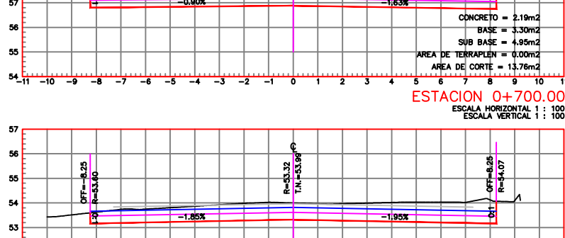
ESTACION 0+700.00 ESCALA HORIZONTAL 1 : 100 ESCALA VERTICAL 1 : 100
