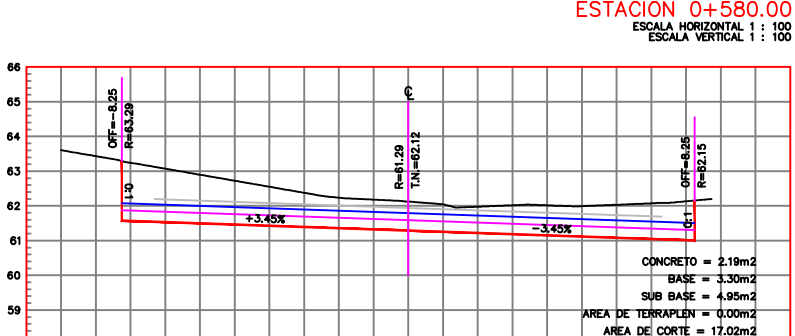
ESTACION 0+600.00 ESCALA HORIZONTAL 1 : 100 ESCALA VERTICAL 1 : 100
