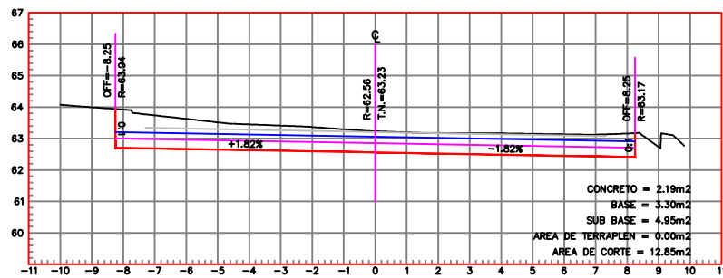
ESTACION 0+640.00 ESCALA HORIZONTAL 1 : 100 ESCALA VERTICAL 1 : 100
