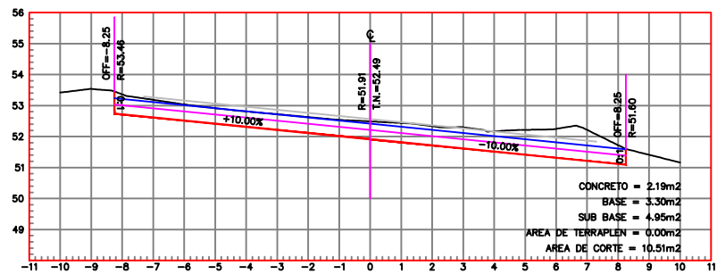
ESTACION 0+440.00 ESCALA HORIZONTAL 1 : 100 ESCALA VERTICAL 1 : 100
