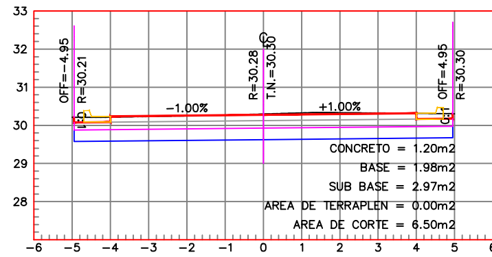
ESTACION 0+095.61 ESCALA HORIZONTAL 1 : 100 ESCALA VERTICAL 1 : 100
