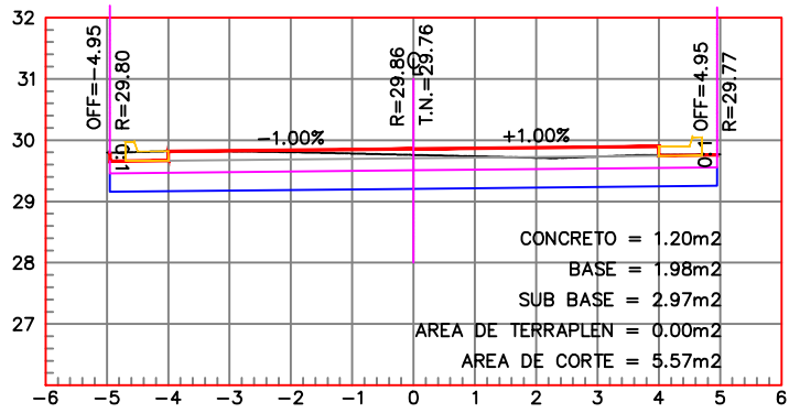
ESTACION 0+040.00 ESCALA HORIZONTAL 1 : 100 ESCALA VERTICAL 1 : 100
