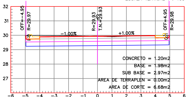
ESTACION 0+050.00 ESCALA HORIZONTAL 1 : 100 ESCALA VERTICAL 1 : 100
