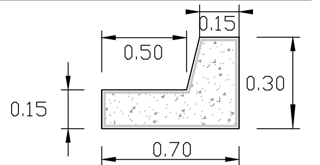
DETALLE DE GUARNICION TIPO "L" (SIN ESCALA)
