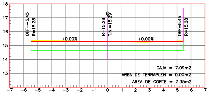
ESTACION 0+060.00
