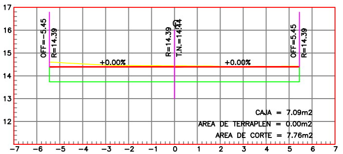
ESTACION 0+090.00
