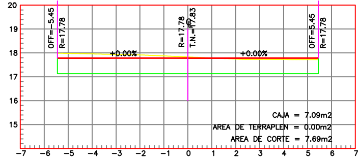
ESTACION 0+010.00
