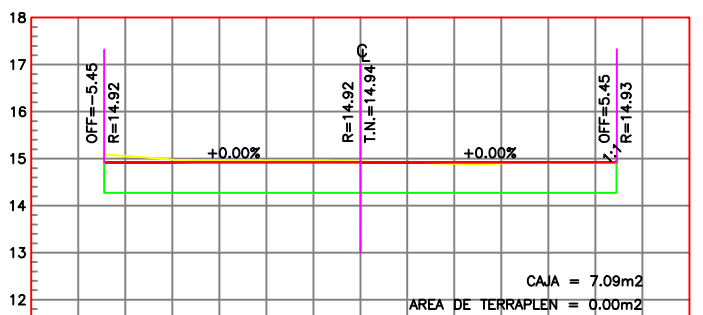
ESTACION 0+070.00
