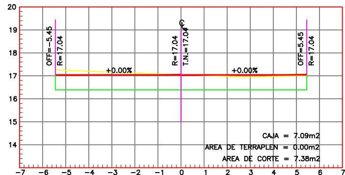
ESTACION 0+020.00
