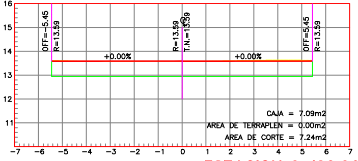
ESTACION 0+128.06
