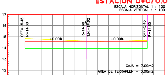
ESTACION 0+080.00
