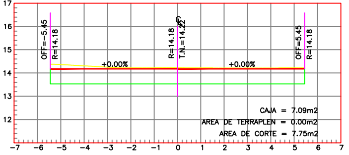
ESTACION 0+100.00
