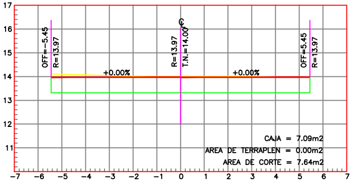
ESTACION 0+110.00
