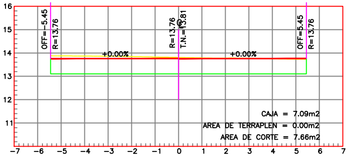
ESTACION 0+120.00
