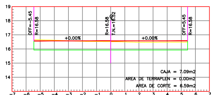
ESTACION 0+030.00
