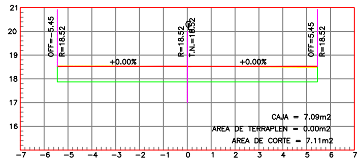
ESTACION 0+000.00
