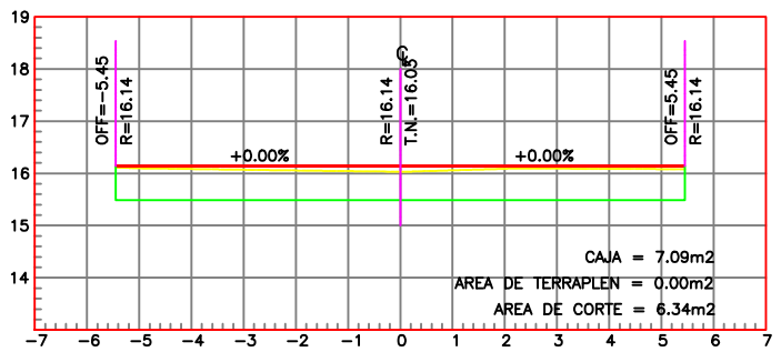
ESTACION 0+040.00
