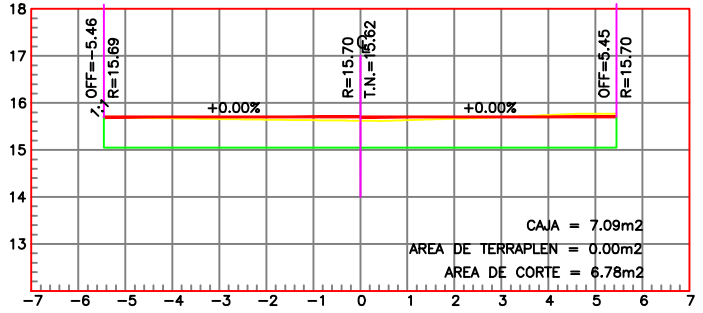
ESTACION 0+050.00
