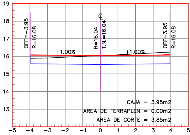
ESTACION 0+200.00
