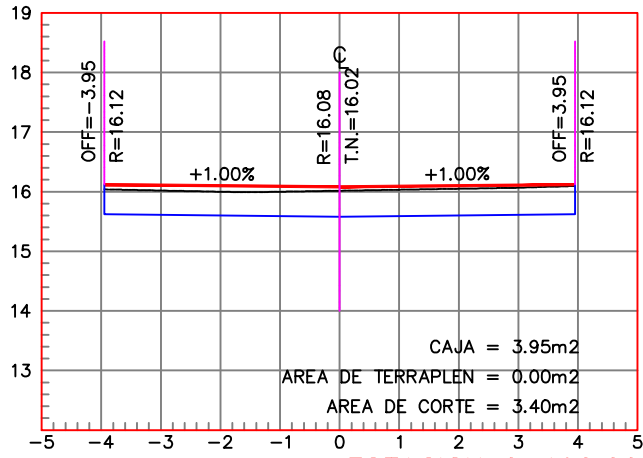
ESTACION 0+190.00
