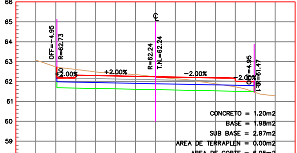
ESTACION 0+090.00 ESCALA HORIZONTAL 1 : 100 ESCALA VERTICAL 1 : 100
