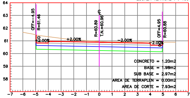
ESTACION 0+040.00 ESCALA HORIZONTAL 1 : 100 ESCALA VERTICAL 1 : 100
