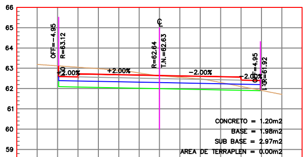
ESTACION 0+100.00 ESCALA HORIZONTAL 1 : 100 ESCALA VERTICAL 1 : 100
