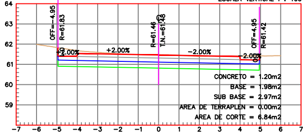
ESTACION 0+060.00 ESCALA HORIZONTAL 1 : 100 ESCALA VERTICAL 1 : 100
