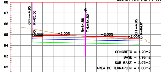
ESTACION 0+160.00 ESCALA HORIZONTAL 1 : 100 ESCALA VERTICAL 1 : 100
