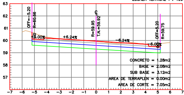
ESTACION 0+010.00 ESCALA HORIZONTAL 1 : 100 ESCALA VERTICAL 1 : 100
