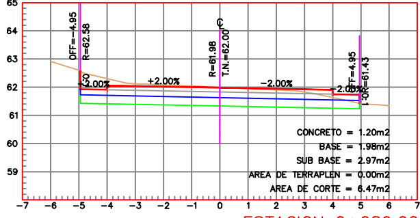
ESTACION 0+080.00 ESCALA HORIZONTAL 1 : 100 ESCALA VERTICAL 1 : 100
