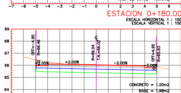
ESTACION 0+190.00 ESCALA HORIZONTAL 1 : 100 ESCALA VERTICAL 1 : 100
