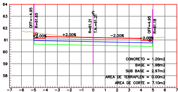
ESTACION 0+050.00 ESCALA HORIZONTAL 1 : 100 ESCALA VERTICAL 1 : 100
