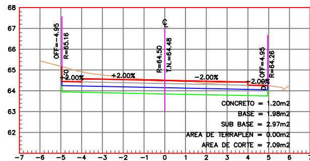
ESTACION 0+150.00 ESCALA HORIZONTAL 1 : 100 ESCALA VERTICAL 1 : 100
