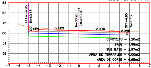
ESTACION 0+020.00 ESCALA HORIZONTAL 1 : 100 ESCALA VERTICAL 1 : 100
