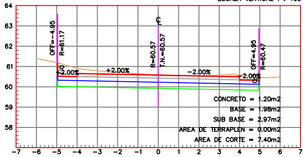
ESTACION 0+030.00 ESCALA HORIZONTAL 1 : 100 ESCALA VERTICAL 1 : 100
