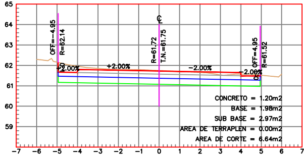
ESTACION 0+070.00 ESCALA HORIZONTAL 1 : 100 ESCALA VERTICAL 1 : 100
