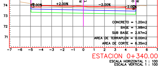
ESTACION 0+340.00 ESCALA HORIZONTAL 1 : 100 ESCALA VERTICAL 1 : 100
