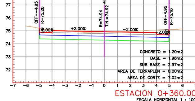
ESTACION 0+360.00 ESCALA HORIZONTAL 1 : 100 ESCALA VERTICAL 1 : 100
