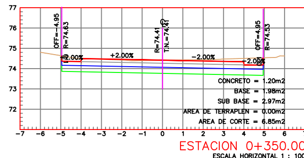
ESTACION 0+350.00 ESCALA HORIZONTAL 1 : 100 ESCALA VERTICAL 1 : 100
