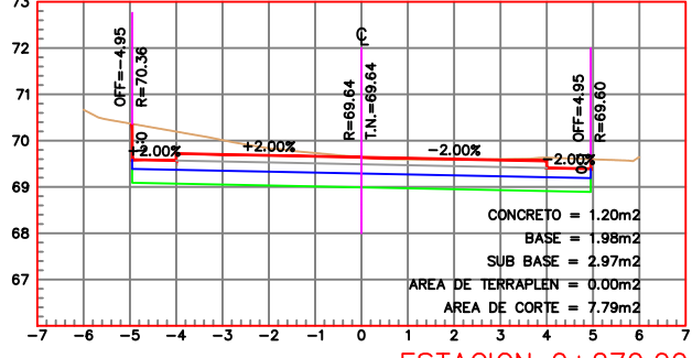
ESTACION 0+270.00 ESCALA HORIZONTAL 1 : 100 ESCALA VERTICAL 1 : 100
