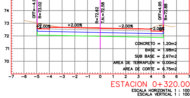
ESTACION 0+320.00 ESCALA HORIZONTAL 1 : 100 ESCALA VERTICAL 1 : 100
