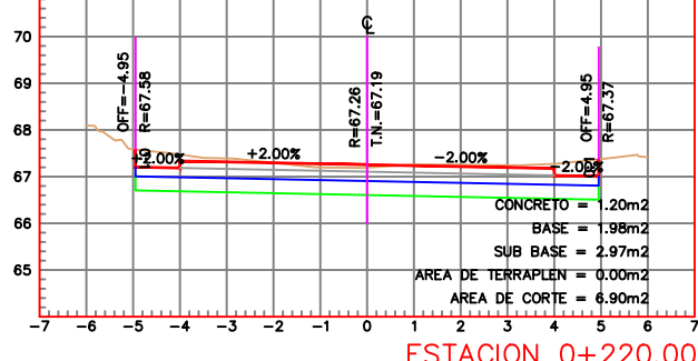
ESTACION 0+220.00 ESCALA HORIZONTAL 1 : 100 ESCALA VERTICAL 1 : 100
