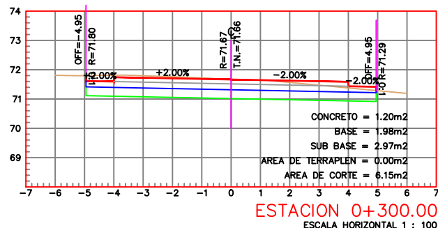
ESTACION 0+300.00 ESCALA HORIZONTAL 1 : 100 ESCALA VERTICAL 1 : 100
