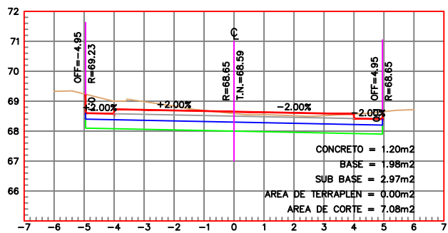
ESTACION 0+250.00 ESCALA HORIZONTAL 1 : 100 ESCALA VERTICAL 1 : 100
