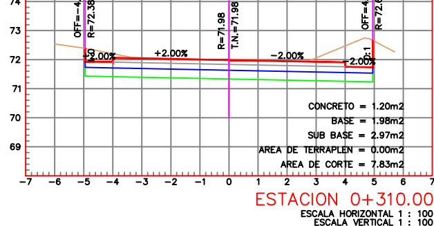
ESTACION 0+310.00 ESCALA HORIZONTAL 1 : 100 ESCALA VERTICAL 1 : 100
