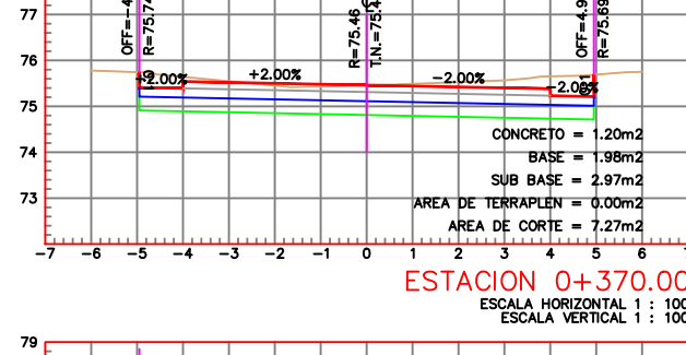
ESTACION 0+370.00 ESCALA HORIZONTAL 1 : 100 ESCALA VERTICAL 1 : 100
