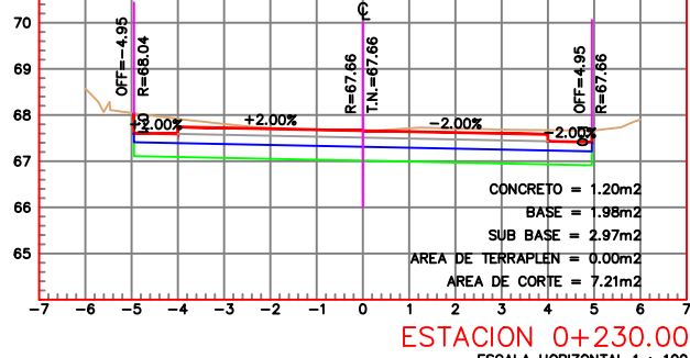
ESTACION 0+230.00 ESCALA HORIZONTAL 1 : 100 ESCALA VERTICAL 1 : 100
