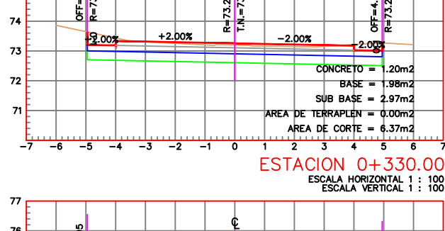
ESTACION 0+330.00 ESCALA HORIZONTAL 1 : 100 ESCALA VERTICAL 1 : 100
