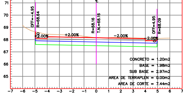
ESTACION 0+240.00 ESCALA HORIZONTAL 1 : 100 ESCALA VERTICAL 1 : 100
