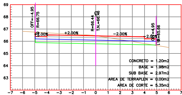
ESTACION 0+200.00 ESCALA HORIZONTAL 1 : 100 ESCALA VERTICAL 1 : 100
