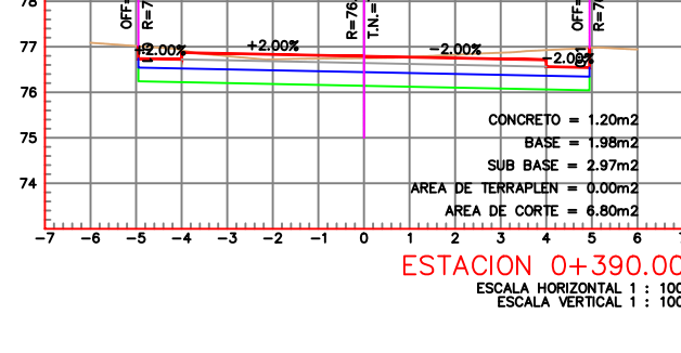
ESTACION 0+390.00 ESCALA HORIZONTAL 1 : 100 ESCALA VERTICAL 1 : 100
