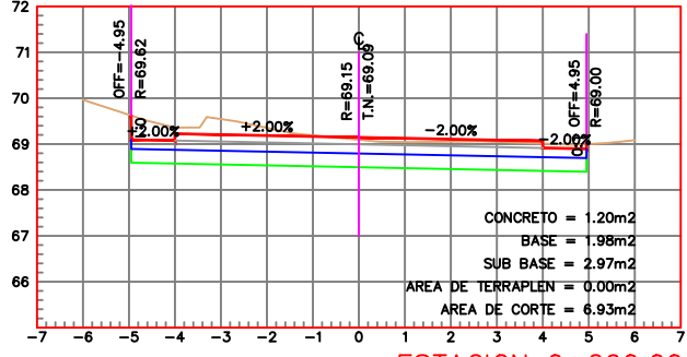
ESTACION 0+260.00 ESCALA HORIZONTAL 1 : 100 ESCALA VERTICAL 1 : 100
