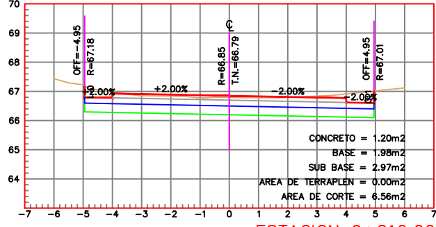
ESTACION 0+210.00 ESCALA HORIZONTAL 1 : 100 ESCALA VERTICAL 1 : 100
