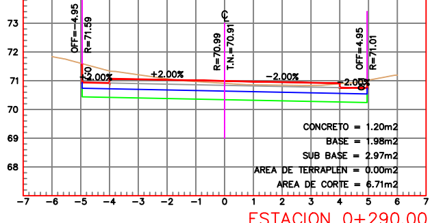
ESTACION 0+290.00 ESCALA HORIZONTAL 1 : 100 ESCALA VERTICAL 1 : 100
