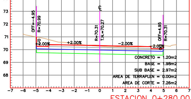
ESTACION 0+280.00 ESCALA HORIZONTAL 1 : 100 ESCALA VERTICAL 1 : 100
