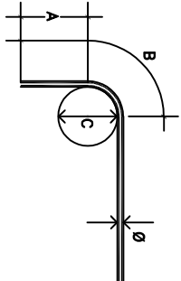
DETALLE DE GANCHOS
