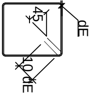
GANCHOS DE ESTRIBOS
