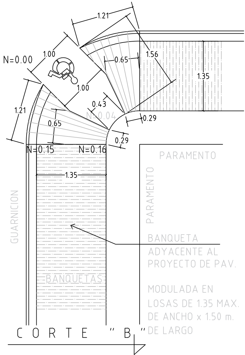
VISTA EN PLANTA DEL DETALLE PARA ACCESO EN BANQUETAS SIN ESCALA
