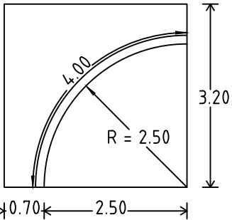
DETALLE DE GUARNICIÓN EN APROCHES (LLEGADAS A CALLES CON PAVIMENTO)
