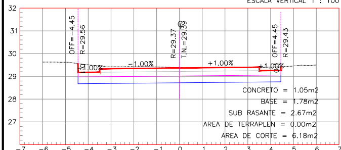
ESTACION 0+010.00
