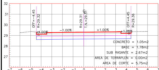
ESTACION 0+000.00
