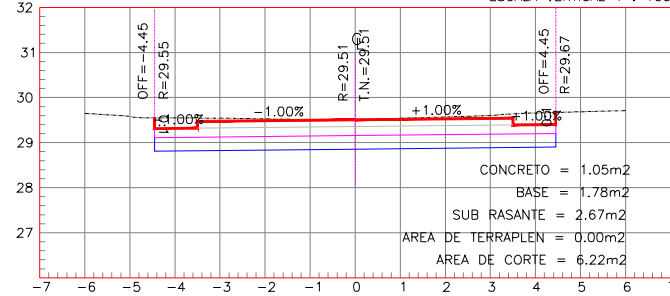
ESTACION 0+110.00
