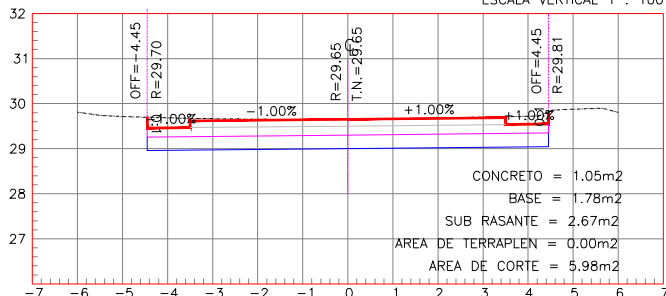
ESTACION 0+060.00
