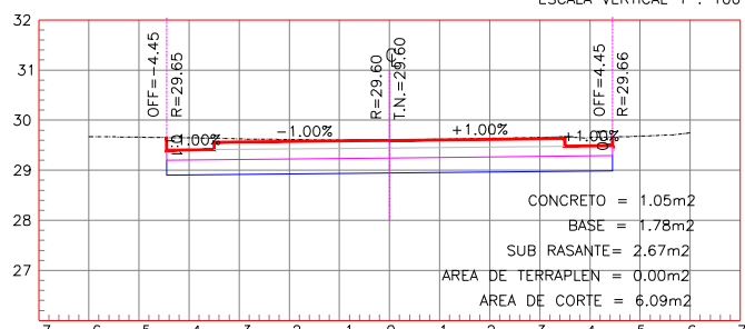
ESTACION 0+050.00
