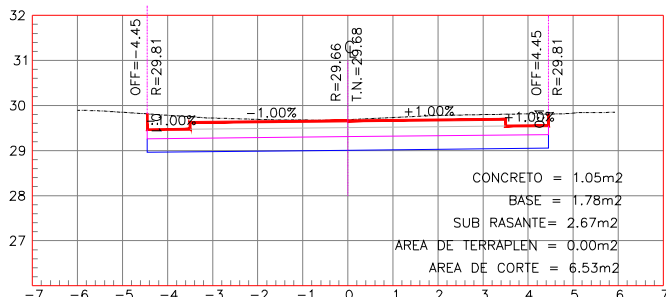
ESTACION 0+080.00
