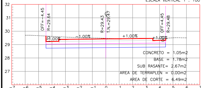
ESTACION 0+020.00
