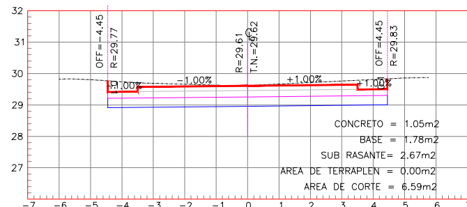
ESTACION 0+090.00
