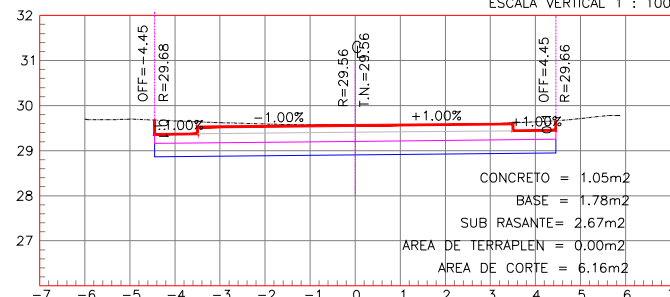
ESTACION 0+100.00
