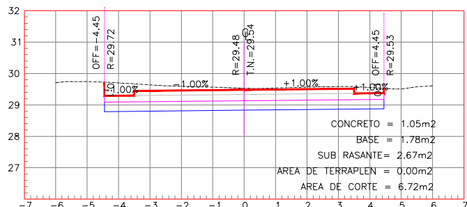
ESTACION 0+030.00
