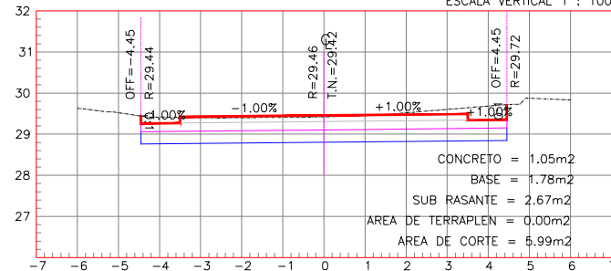
ESTACION 0+120.00
