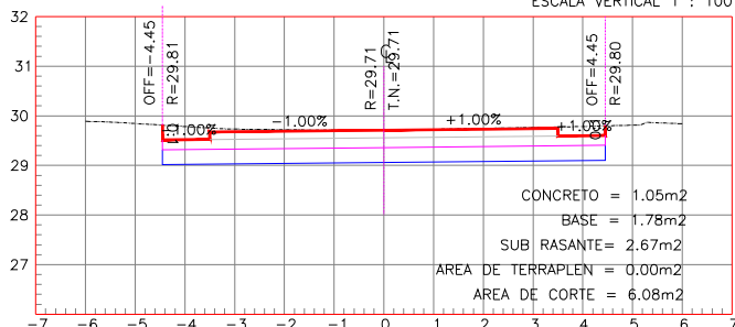
ESTACION 0+070.00
