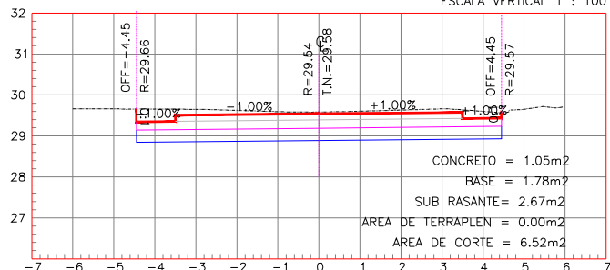
ESTACION 0+040.00
