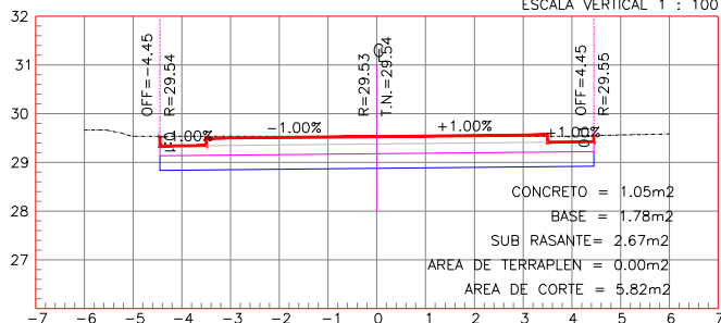
ESTACION 0+180.00
