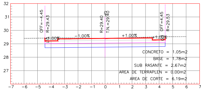
ESTACION 0+130.00
