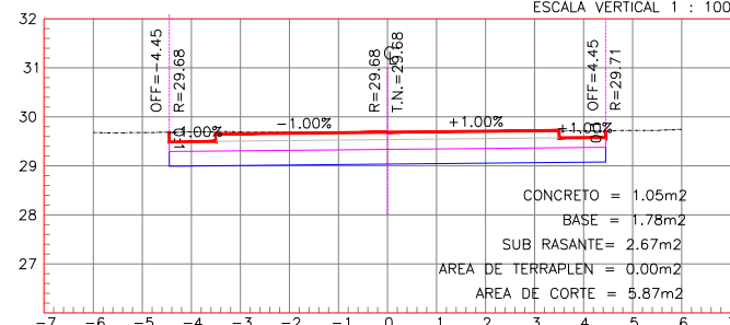
ESTACION 0+240.00
