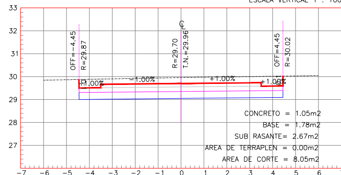
ESTACION 0+245.98
