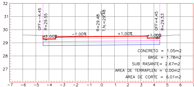
ESTACION 0+160.00
