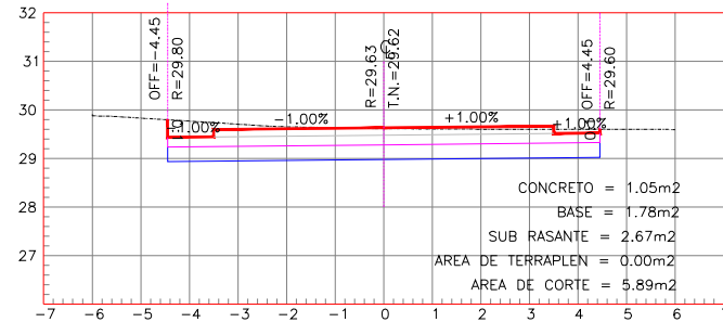
ESTACION 0+220.00
