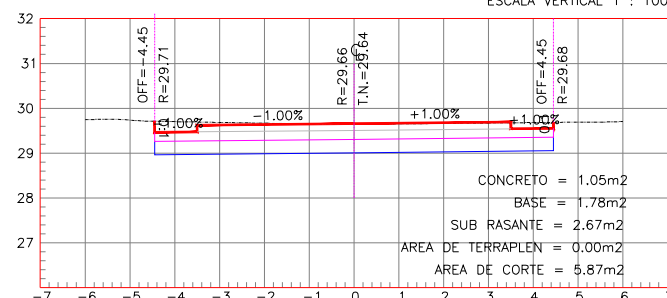
ESTACION 0+230.00
