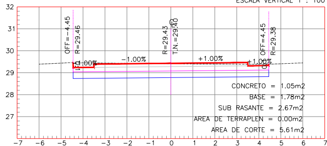
ESTACION 0+140.00
