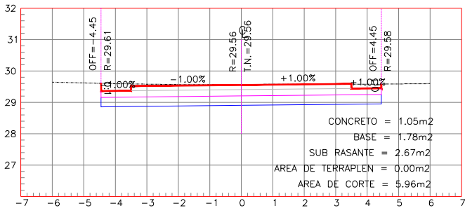
ESTACION 0+190.00
