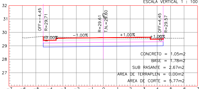
ESTACION 0+210.00
