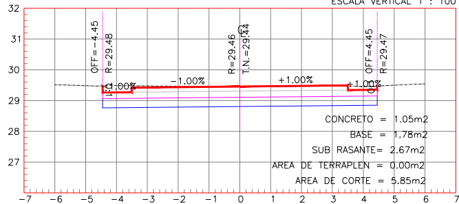
ESTACION 0+150.00
