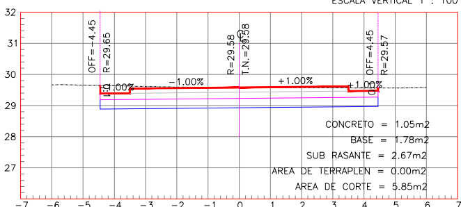
ESTACION 0+200.00
