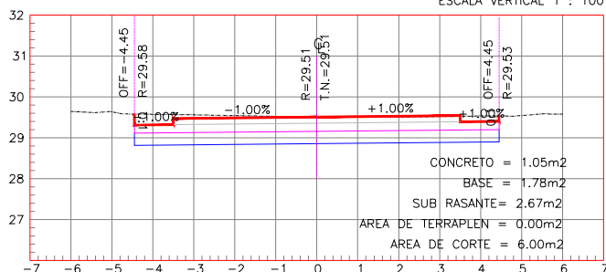
ESTACION 0+170.00
